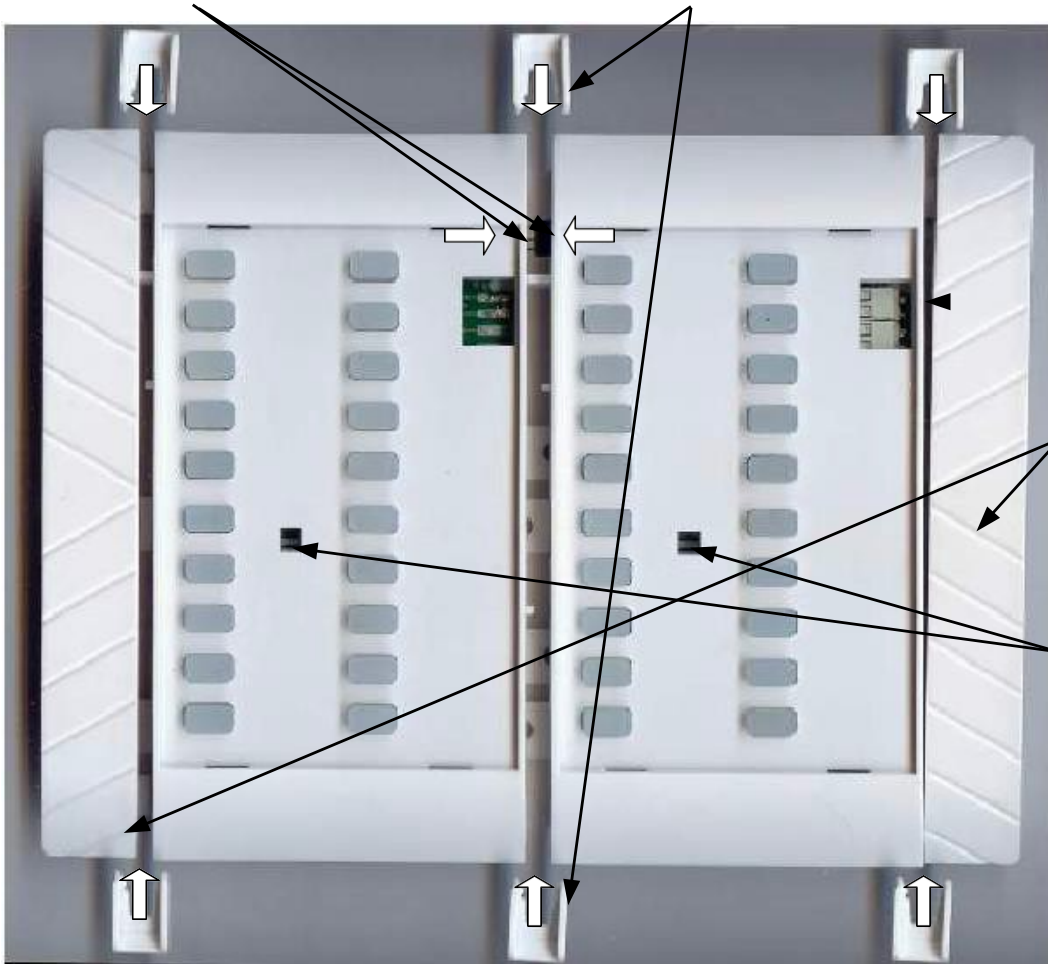
Рис. 8 Сборка блоков БИС-М и БИС-М1
