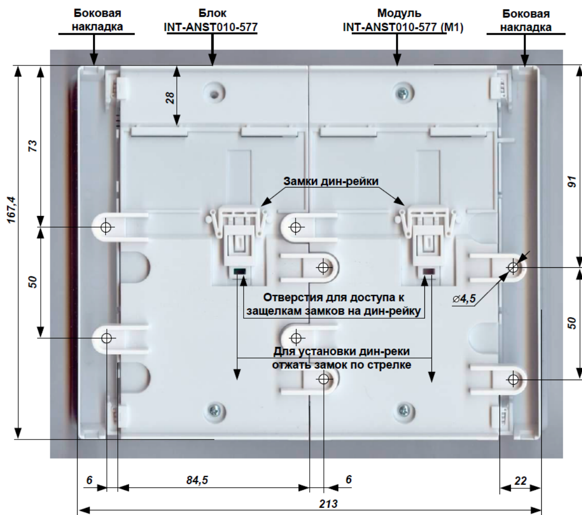
Рис. 4 Вид сзади. Габаритные и присоединительные размеры.
